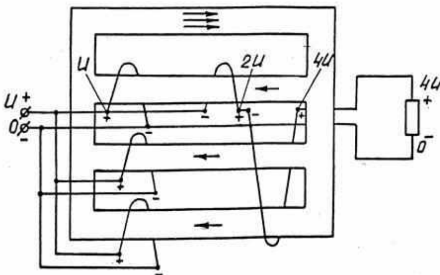
Рисунок 1 – Импульсный трансформатор
